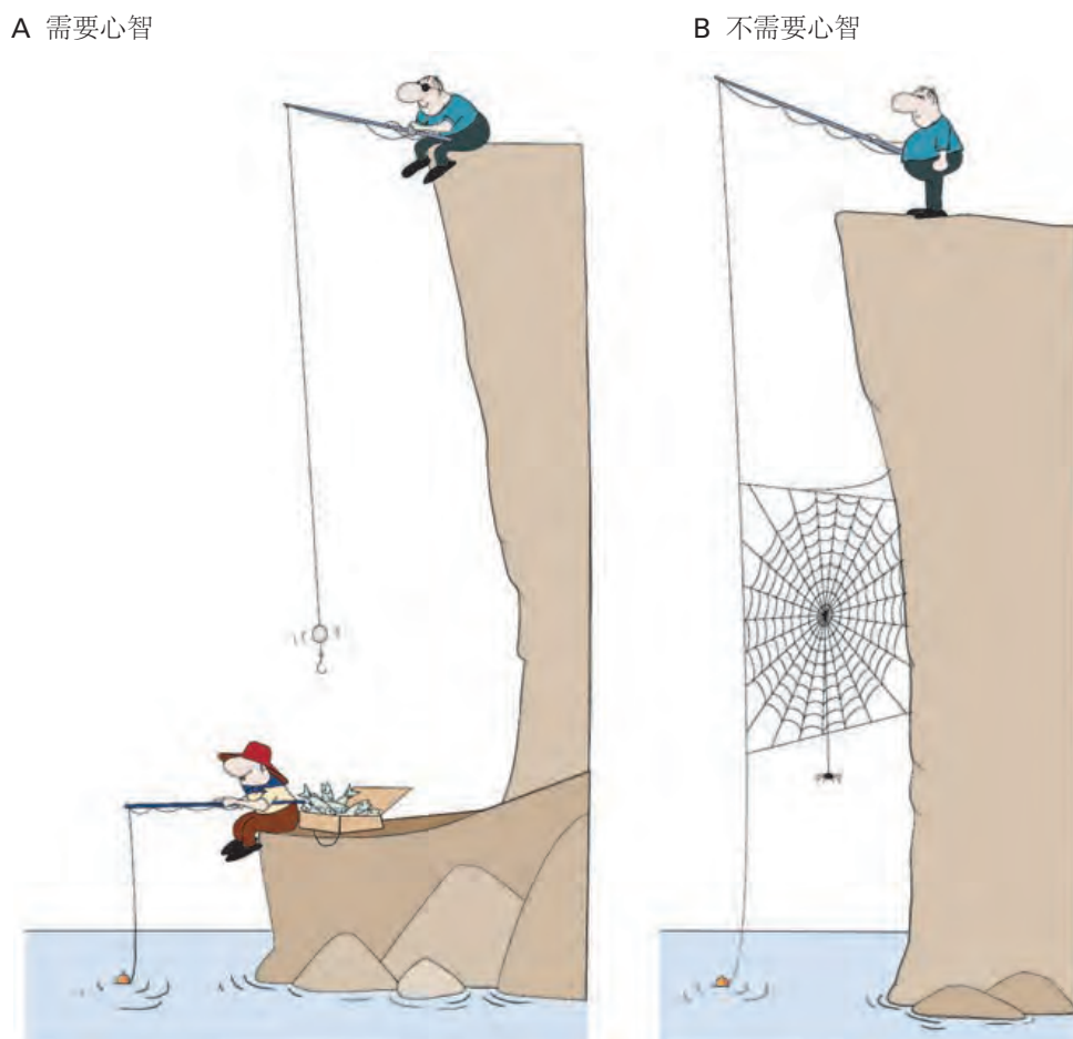
图 62.2.3: 用于“心智化”成像研究的卡通示例。要求参与者（静默地）考虑每张图片的含义，然后对其进行解释。在一项功能性核磁共振成像研究中，正常成年人被动观看需要心智化的卡通片和不需要心智化的卡通片。如图 62.2.4 所示，每个受试者的大脑区域特征网络都被激活 [553] 。
