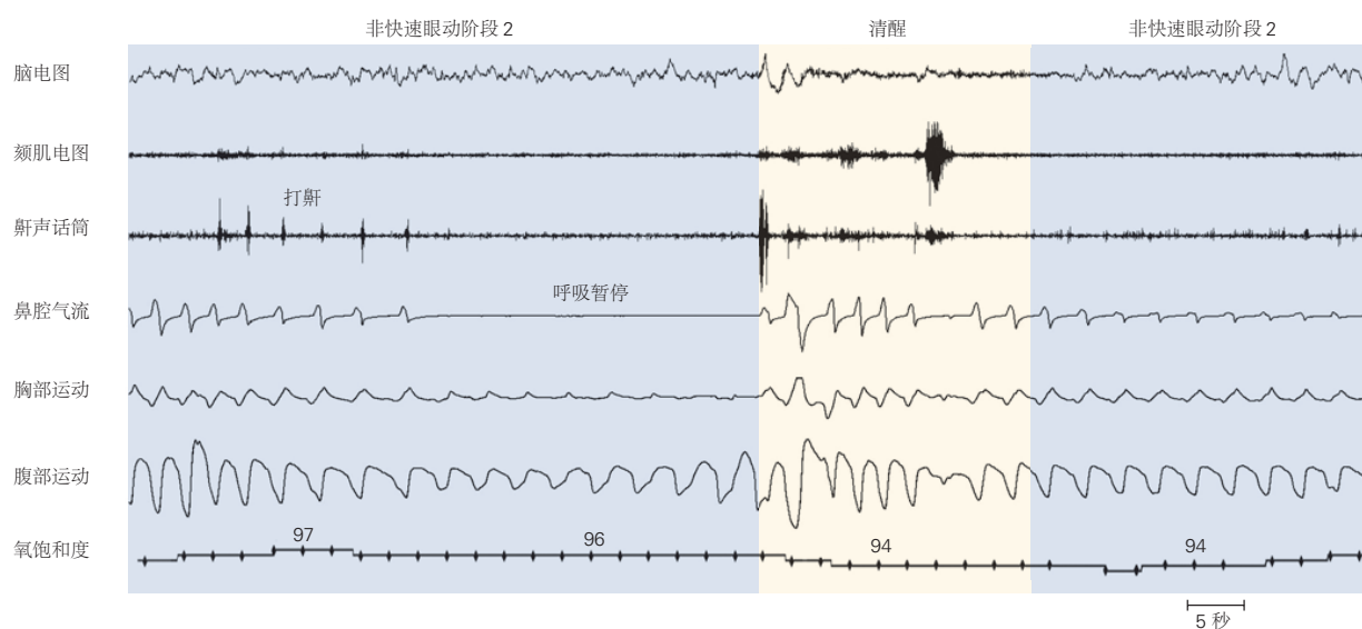
图 44.5.1: 睡眠呼吸暂停发作。在这个多导睡眠图的开始，一个人处于非快速眼动阶段 2 睡眠。检测到一些打鼾，但鼻腔气流良好且氧饱和度正常。然后，个体会出现阻塞性呼吸暂停，没有鼻腔气流；然而，呼吸努力仍然存在（由腹部运动显示）。呼吸暂停由短暂的觉醒（低电压快速脑电图）终止，伴随着响亮的鼾声、肌电图活动增加、呼吸努力增强和气道开放。氧饱和度下降约 3%，在呼吸暂停结束约 15 秒后达到最低点，因为血液从肺部流到测量氧饱和度的指尖需要时间。
