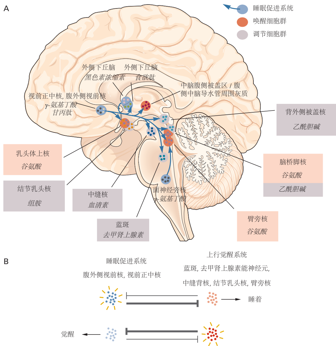
图 44.2.2: 促进睡眠的通路。 A. 如图 44.2.1 所示，上行觉醒系统的组成部分从促进睡眠的神经元接收抑制性的、主要是 \gamma -氨基丁酸能的输入。腹外侧视前核和视前正中核中的神经元支配整个觉醒促进系统，而面神经旁核中的神经元主要支配臂旁区域。许多腹外侧视前核神经元还含有甘丙肽（一种抑制肽）。如图 44.2.3 所示，外侧下丘脑中释放黑色素浓缩素的神经元可通过抑制附近的食欲能神经元以及导水管周围灰质中阻止快速眼动睡眠的神经元来促进快速眼动睡眠。B. 腹外侧视前核和正中视前核与上行觉醒系统相互抑制成分的触发器开关关系。当被激活时，促进睡眠的神经元会抑制上行觉醒系统的组成部分。然而，促进睡眠的细胞群也受到觉醒系统的抑制。最终效果是个人大部分时间都处于完全觉醒或睡眠状态，同时最大限度地减少过渡状态的时间。
