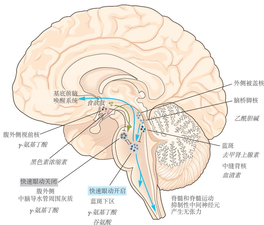
图 44.2.3: 快速眼动睡眠开关。脑干神经元对于控制非快速眼动和快速眼动睡眠之间的转换至关重要。快速眼动睡眠是由脑桥头端的一群神经元产生的，就在背侧被盖核和蓝斑的腹侧，在啮齿动物中称为亚侧背区，在人类中称为蓝斑下区。这些谷氨酸能神经元投射到脑干的其他部分，在那里它们启动快速眼动睡眠的运动和自动表现，并投射到前脑，在那里它们调节快速眼动睡眠的行为和脑电图成分。下行投射激活延髓和脊髓中的抑制性中间神经元，使运动神经元极化并阻止个体实现他梦中所想。如图 44.2.2B 所示，这些快速眼动开启神经元被腹外侧导水管周围灰质和邻近的脑桥网状结构中的 \gamma -氨基丁酸能神经元抑制，而后者本身被快速眼动开启区域的神经元抑制，从而形成触发器开关。这些快速眼动关闭神经元受前脑神经元控制，包括释放兴奋性食欲素神经肽的神经元、释放抑制性信号分子 \gamma -氨基丁酸和甘丙肽的腹外侧视前核神经元，以及释放抑制性神经肽黑色素浓缩素的下丘脑神经元。此外，蓝斑和中缝背侧的调节神经元会抑制快速眼动生成器，而脑桥脚核和背侧被盖核中的胆碱能神经元会促进快速眼动睡眠。该模型解释了许多临床观察结果，例如胆碱能激动剂药物促进快速眼动睡眠，而增加单胺水平的抗抑郁药等药物抑制快速眼动睡眠。食欲素神经元的缺失会导致快速眼动睡眠突然开始，而背侧下区域的快速眼动启动神经元缺失会消除快速眼动睡眠期间的张力缺失。因此，患有这种疾病的人会在梦中表演（快速眼动睡眠行为障碍）。
