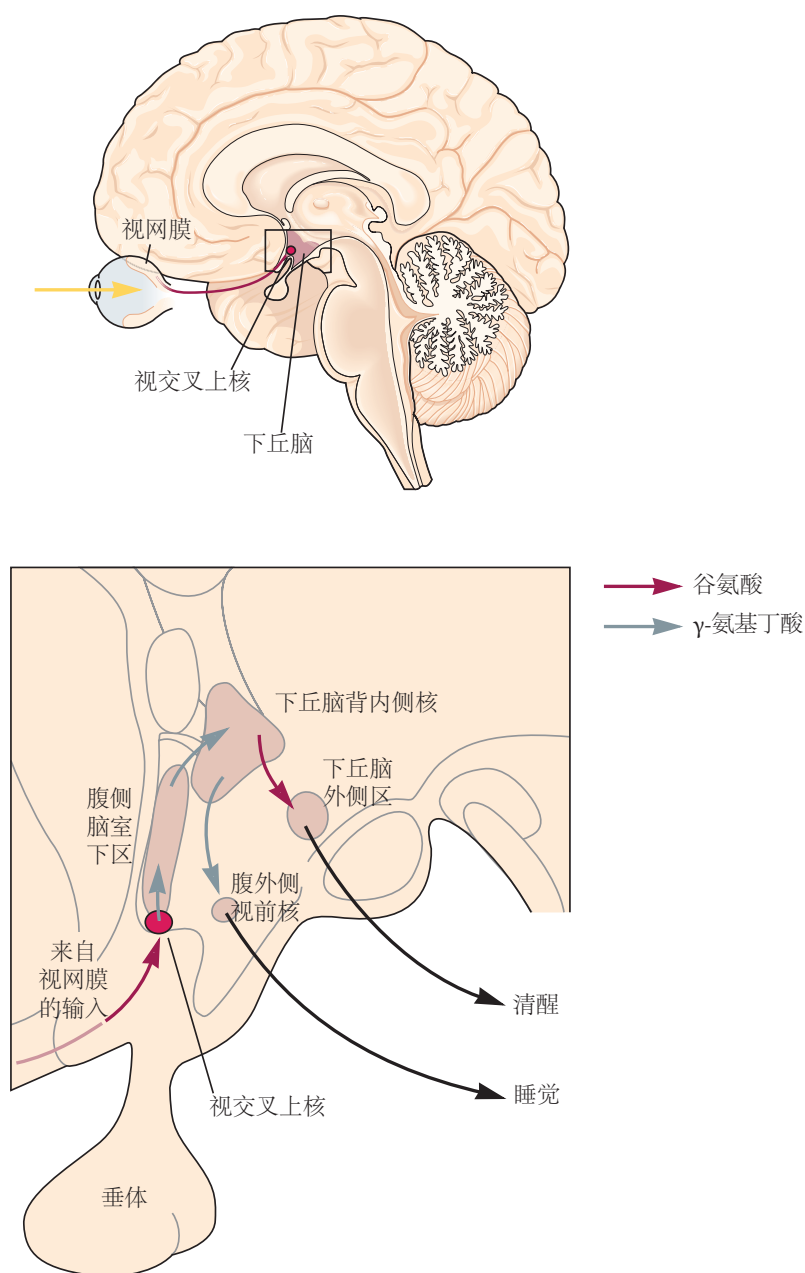
图 44.3.2: 视交叉上核中的神经元为觉醒-睡眠提供了一个主时钟。视网膜输入光信号激活视交叉上核（上图），然后通过下丘脑中的一系列转发器驱动唤醒-睡眠周期（下图）。通过下丘脑的矢状切面显示视交叉上核投射到腹侧脑室下区中的神经元，后者又投射到下丘脑背内侧核。下丘脑背内侧核含有谷氨酸能神经元，可刺激下丘脑外侧区中的食欲能神经元和谷氨酸能神经元，从而引起觉醒。下丘脑背内侧核中的 \gamma -氨基丁酸能神经元会抑制腹外侧视前核，从而关闭促进睡眠的系统。患有下丘脑背内侧核病变的动物无法表现出昼夜节律，每天多睡一个小时左右。
