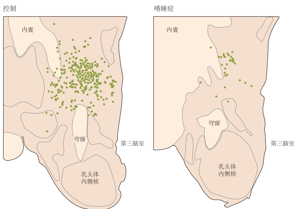
图 44.5.2: 发作性睡病与产生食欲素神经肽的下丘脑神经元的丧失有关。与正常大脑（左）相比，患有发作性睡病（右）的个体在乳头体水平的大脑截面图中可以明显看出食欲神经元（绿点）的明显丧失 [380] 。
