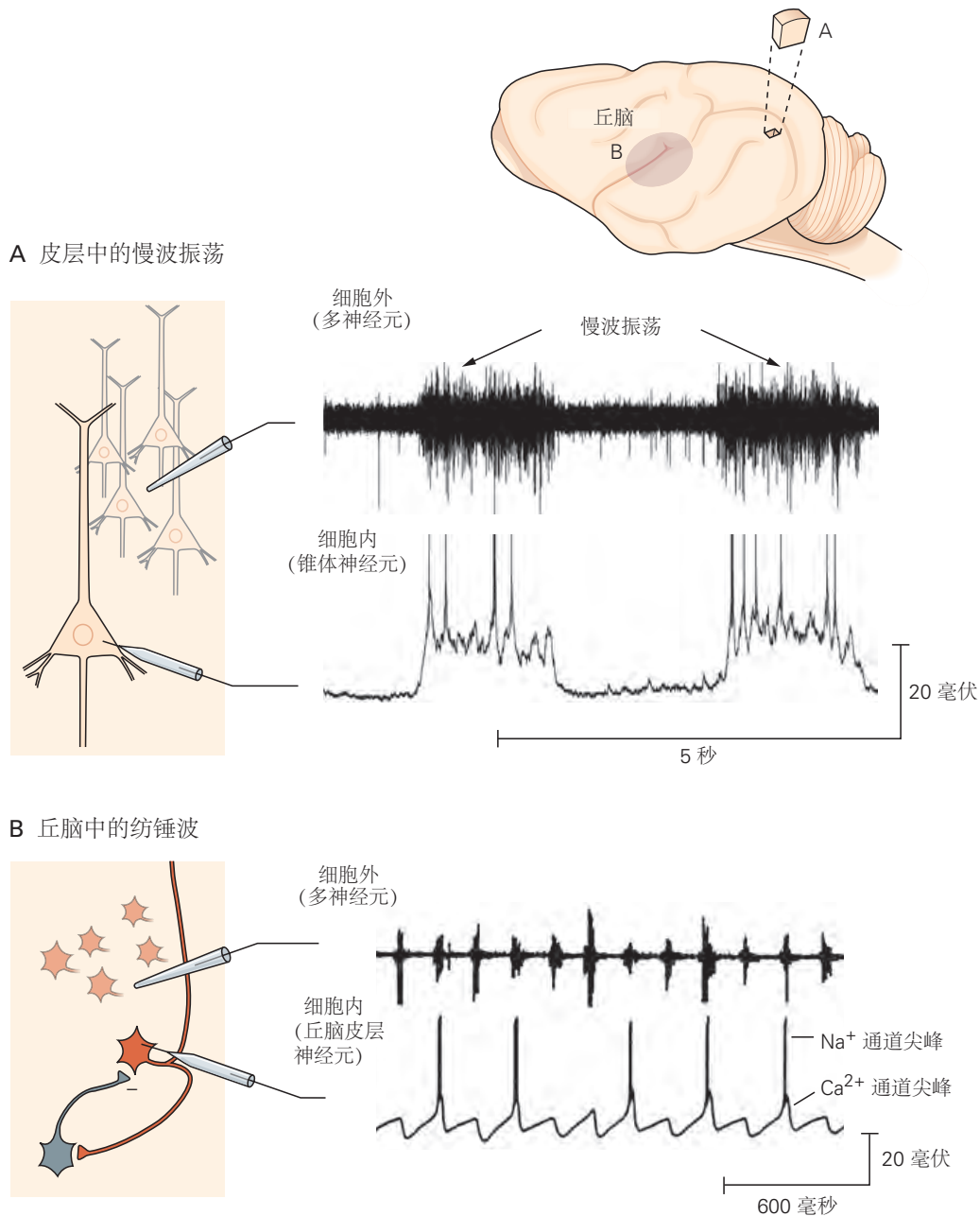
图 44.1.1: 睡眠期间脑电图节律的细胞机制。A. 在非快速眼动睡眠期间构成脑电图慢波基础的慢波振荡是由大脑皮质内在的大量反复兴奋连接和抑制连接产生的。即使在孤立的皮质板中，慢波也会继续。当单个神经元超极化并且不放电时，来自此类神经元的细胞内记录在缓慢振荡期间显示有节奏的向下状态，当膜电位去极化更多并且神经元激发多个动作电位时与向上状态交替。这种同步放电会产生树突状电位波，在脑电图中表现为慢波。B. 同样，在丘脑切片中，循环回路产生纺锤波。网状核神经元（灰色）中的脉冲使丘脑皮层中继神经元（红色）超极化，足以使低阈值（T 型）Ca 2+ 通道失活。随着超极化减弱，这些 Ca 2+ 通道打开，由此产生的 Ca 2+ 电流使中继神经元去极化，在 Ca 2+ 通道脉冲平台顶部产生短暂的 Na + 通道脉冲。同时，随着中继细胞的持续爆发，其兴奋性输出在网状神经元中产生 T 型 Ca 2+ 通道脉冲，从而驱动另一次 Na + 脉冲爆发。由此产生对中继细胞的反馈抑制启动了一个新的爆发周期。这种放电模式每秒重复 12 到 14 次，由此产生的到达皮层的丘脑皮层动作电位波在脑电图中产生睡眠纺锤波。上部迹线显示了本地中继细胞群的动作电位。下部迹线显示抑制性突触后电位和来自单个中继细胞的脉冲；在这个缓慢的时间基础上，细胞内记录中的每个上行代表最多 6 个动作电位的爆发。正如轨迹所示，在纺锤波的每个周期中，单个中继神经元都不会达到脉冲阈值。因此，细胞外脉冲活动的幅度因周期而异，这取决于恰好激发哪些神经元以及它们与细胞外电极尖端的距离。然而，每次丘脑放电的爆发都会在皮质中产生一连串兴奋性突触后电位，从而导致脑电图波与丘脑放电时间锁定 [379] 。
