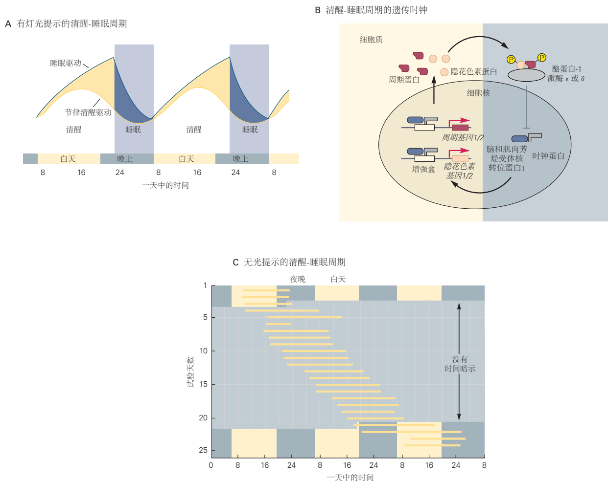
图 44.3.1: 觉醒的昼夜节律驱动力与睡眠的稳态驱动力相互作用，形成觉醒-睡眠周期。A. 睡眠内驱力在长时间觉醒的过程中逐渐增强，而昼夜节律内驱力以 24 小时为周期变化，与之前的睡眠无关。这种昼夜节律觉醒周期的高峰出现在睡前几个小时，因为稳态睡眠驱动正在上升，而低点出现在习惯性觉醒时间之前的几个小时，此时睡眠的稳态驱动正在减弱。B. 哺乳动物细胞的 24 小时节律由一组形成转录-翻译环的蛋白质调节。脑和肌肉芳烃受体核转位蛋白 1 和时钟蛋白形成一个二聚体，与许多具有昼夜节律转录的基因上发现的增强盒基序结合。其中包括周期基因 1 和周期基因 2 和隐花色素基因 1 和隐花色素基因 2。他们的产物二聚化并与酪蛋白-1 激酶 \epsilon 或 \delta 形成复合物。该复合物易位至细胞核，在那里它抑制脑和肌肉芳烃受体核转位蛋白 1 和时钟蛋白的二聚化，导致它从增强盒脱落。这减少了周期基因和隐花色素基因的转录；随着周期蛋白和隐花色素蛋白的降解，脑和肌肉芳烃受体核转位蛋白 1 和时钟蛋白再次二聚化，然后循环重复。C. 昼夜节律调节睡眠和觉醒的时间。该图显示了一个人的觉醒周期（黄色条），他最初在正常照明条件下生活了 3 天，然后在没有时间线索的昏暗环境中生活了 18 天。个体每天维持约 25.2 小时的周期，在此期间漂移一整天。如图 44.3.2 所示，无法将光信号传递到视交叉上核的盲人经常像这样连续生活，这种情况称为非 24 小时觉醒睡眠障碍。
