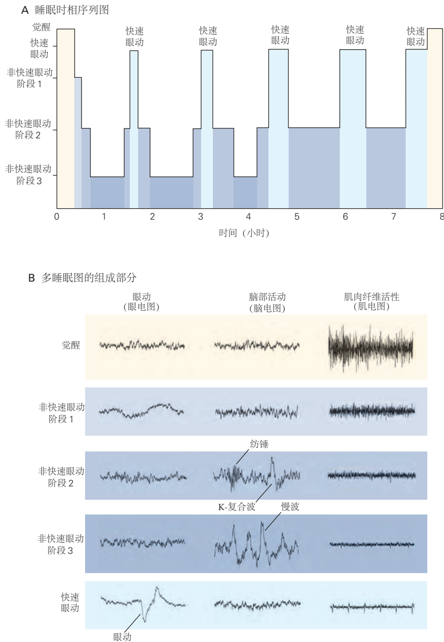
图 44.0.1: 觉醒和睡眠的电生理模式。A. 一张睡眠时相序列图或图表，显示健康年轻人在典型夜晚的睡眠阶段进展。快速眼动睡眠周期与非快速眼动睡眠周期大约每 90 分钟交替一次。一个人通常会从觉醒状态进入浅度非快速眼动阶段 1 睡眠，然后逐渐进入更深的非快速眼动睡眠（非快速眼动阶段 2、非快速眼动阶段 3），然后在第一阶段快速眼动睡眠发生之前回到较浅的非快速眼动睡眠（浅蓝色条）。随着夜晚的推移，个体在非快速眼动睡眠的最深阶段花费的时间越来越少，而快速眼动睡眠期的持续时间会增加。B. 记录显示用于区分睡眠阶段的多导睡眠图的组成部分。眼电图通过眼睛两侧的电极记录眼球运动。脑电图记录头皮的皮层场电位；肌电图记录通过皮肤的肌肉纤维放电。在觉醒状态下，眼电图显示自主眼球运动，脑电图显示快速低振幅活动，肌电图显示可变肌张力。非快速眼动阶段 1 睡眠的特点是脑电图频率略有减慢，眼球运动缓慢，肌电图活动较少；非快速眼动阶段 2 的特点是爆发 12 至 14 赫兹的活动，称为睡眠纺锤波和称为 K 复合波的高压慢波；非快速眼动阶段 3 以高压慢波为主。在快速眼动睡眠期间，脑电图与觉醒状态相似。在眼电图上可以看到快速的眼球运动，但肌电图非常安静，有时可以看到微小的心电图信号的污染（如图所示）。
