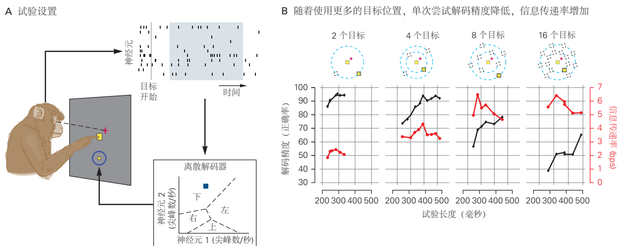
图 39.3.1: 交流脑机接口可以使用基于准备时期神经活动的离散解码器来控制计算机光标。A. 当一只猴子触摸到一个中心目标（黄色大方块）并注视一个中心点（红色+）后，出现了一个外围目标（黄色小方块），猴子准备伸手去拿。脉冲计数是在准备时期进行的，并被输入到一个离散的解码器中。脉冲计数的持续时间（即浅蓝色阴影的宽度）会影响解码性能和信息传递率（参见面板 B）。根据脉冲计数（蓝色方块），离散解码器猜测猴子准备到达的目标。B. 针对不同的试验长度和目标数量显示解码精度（黑色）和信息传递率（比特/秒；红色）。试验长度等于脉冲计数的持续时间（在实验期间变化）加上 190 毫秒（在实验期间固定）。后者提供了外围目标的视觉信息到达前运动皮层的时间（150 毫秒），加上从神经活动中解码目标位置并在屏幕上呈现解码目标位置的时间（40 毫秒） [352] 。
