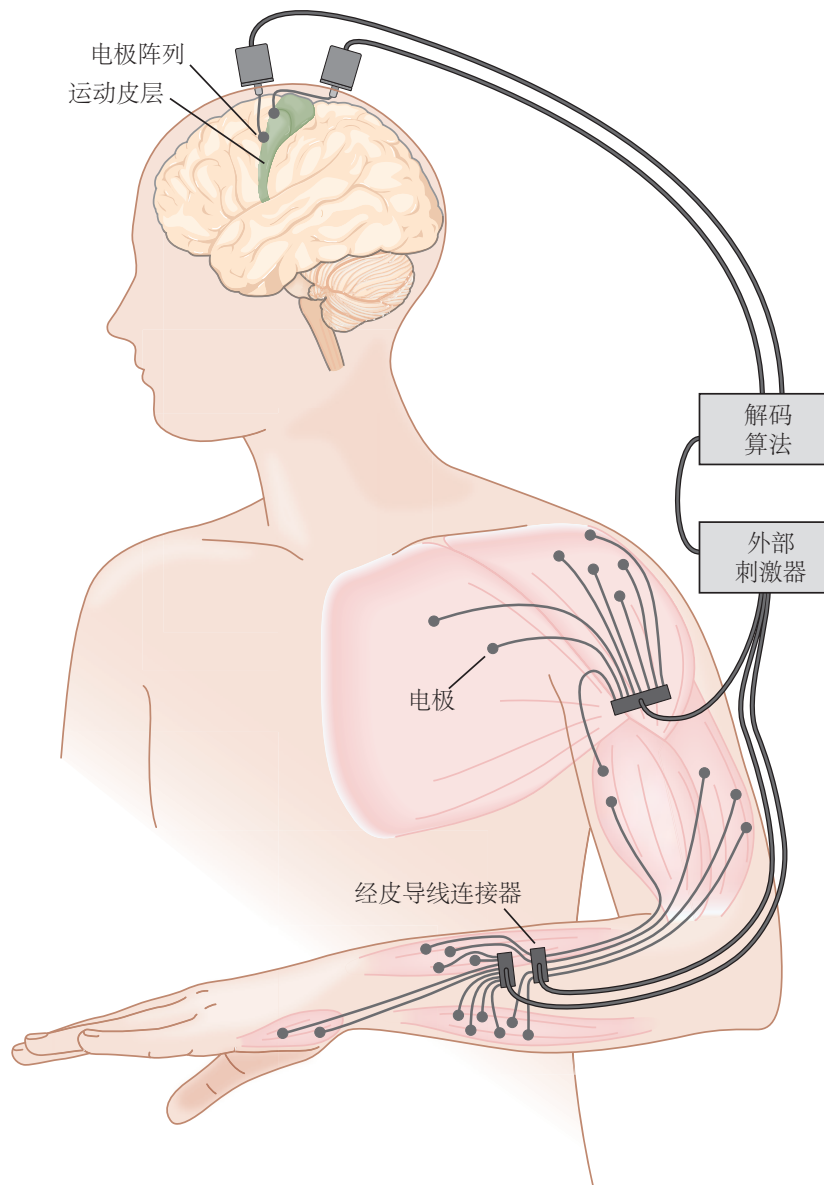
图 39.3.5: 运动脑机接口可以使用连续解码器和功能性电刺激来控制瘫痪手臂的肌肉。将运动皮层中记录的神经活动解码为控制三角肌、胸大肌、二头肌、三头肌、前臂和手部肌肉刺激的命令信号。这使得皮层能够控制整个手臂的运动和抓握。肌肉刺激是通过经皮肌内细线电极进行的 [357] 。
