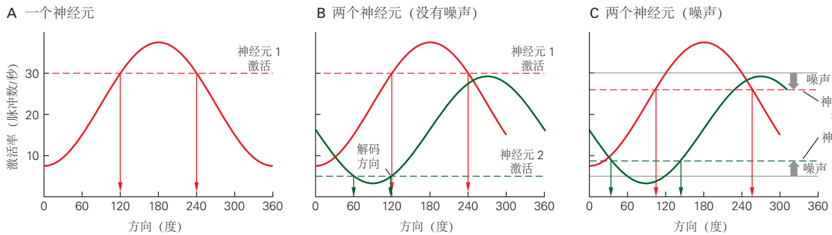
图 39.2.2: 准确的运动解码需要不止一个神经元。A. 一个神经元的调谐曲线定义了神经元的活动如何随运动方向变化。如果此神经元显示 30 个脉冲/秒的活动，则它可能对应于 120^\circ 或 240^\circ 方向的运动。B. 具有不同调谐曲线的第二个神经元（绿色）显示 5 个脉冲/秒的活动，这可能对应于 60^\circ 或 120^\circ 方向的运动。唯一与 2 个神经元的活动一致的运动方向是 120^\circ ，这被确定为解码方向。C. 因为神经活动是“嘈杂的”（表示为虚线的垂直位移），通常不可能从 2 个神经元的活动中最终确定运动方向。在这里，没有一个运动方向与 2 个神经元的活动一致。
