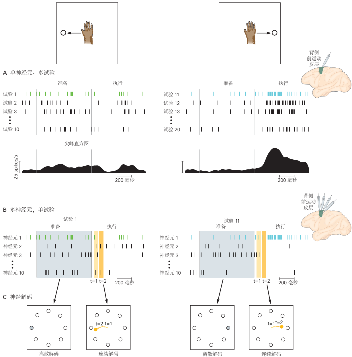
图 39.2.1: 运动编码使用在实验性试验中平均的单个神经元的活动，而运动解码使用单个实验性试验中许多神经元的活动。 A. 准备和执行左臂运动（左）和右臂运动（右）的猴子背侧前运动皮层中记录的一个神经元的活动。表征神经元的运动编码涉及确定神经元在重复向左或向右运动（每行脉冲序列）中的活动如何与手臂运动的各个方面相关。下面是这个神经元向左和向右运动的脉冲直方图，通过对试验中的神经活动进行平均获得。该神经元显示出更高水平的向左运动准备活动和更高水平的向右运动执行活动。背侧前运动皮层和初级运动皮层中的许多神经元在准备和执行时期都显示出与运动相关的活动，就像所示的神经元一样。 B. 背侧前运动皮层记录的许多神经元活动，一次向左运动（左）和一次向右运动（右）。神经元 1 的脉冲序列对应于 A 部分中所示的脉冲序列。脉冲计数是在准备时期进行的，通常在 100 毫秒或更长的大时间段内进行，以估计运动目标。相比之下，脉冲计数在执行时期通常在许多较小的时间段中进行的，每个时间段持续数十毫秒。使用如此短的时间段提供了估计运动的每时每刻细节所需的时间分辨率。 C. 神经解码涉及在单个实验性试验中从许多神经元中提取运动信息。在受试者的工作空间中，有 8 个可能的目标（圆圈）。如图 39.2.3 所示，离散解码提取目标位置；估计的目标用灰色填充。相反，如图 39.2.4 所示，连续解码提取运动的每时每刻的细节；橙色点代表某一时刻的估计位置。
