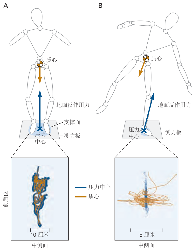
图 36.1.1: 通过移动压力中心来控制质心。A. 重力引起的力通过躯干中的质心。表面对每只脚施加向上的力，使得地面反作用力向量起源于支撑表面上的压力中心。下图：即使脚保持原位，压力中心（蓝色位移）和质心（金色位移）也会随着我们摇摆而运动。在双脚正常站立期间，身体质心的投影保持在支撑底部（与地面接触脚周围的浅蓝色矩形）内以达到平衡。站立的人的支撑基础由脚在支撑表面上的接触来定义。B. 在动态情况下，例如单腿站在窄梁上，即使身体质心位移（黄金位移）短时间超出支撑底部，也可以保持平衡。上下半身反向旋转等策略可以倾斜地面反作用力，从而使身体质心加速回到其支撑基础之上 [328] 。
