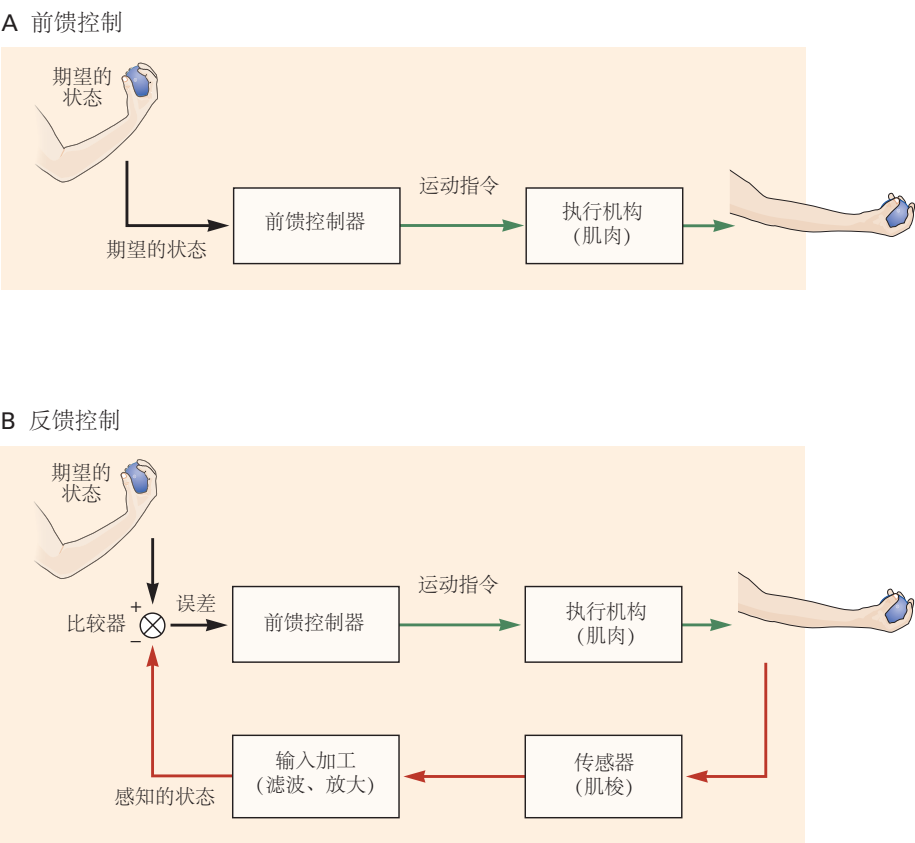
图 30.4.1: 前馈和反馈控制。A. 前馈控制运动命令基于所需状态。不会监控移动过程中出现的误差。虽然我们说明了手臂前馈控制的元素，但只有任何手臂运动的初始部分是由前馈信号驱动的，并且运动通常涉及反馈控制。B. 通过反馈控制，比较所需状态和感测状态（在比较器处）以生成误差信号，这有助于形成运动命令。感觉信息反馈给比较器可能会有相当大的延迟。
