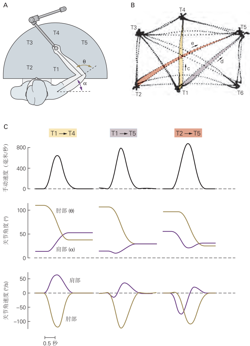
图 30.5.1: 手的路径和速度具有定型特征 [252] 。A. 受试者坐在一个半圆形板前，抓住一个在水平面上移动并记录手部位置的双关节装置的手柄。指示受试者在各种目标 (T1–T6) 之间移动手。B. 一个对象在目标之间移动他的手时所追踪的路径。C. 面板 B 中显示的 3 个手部路径 (c、d 和 e) 的运动学数据。所有路径大致都是直的，并且所有手部速度曲线具有相同的形状和比例，与覆盖的距离成比例。相比之下，3 个手部路径的肘部和肩部角速度分布不同。笔直的手部路径和速度的通用配置文件表明，规划是参考手部完成的，因为这些参数可以线性缩放。参考关节进行规划需要计算关节角度的非线性组合。
