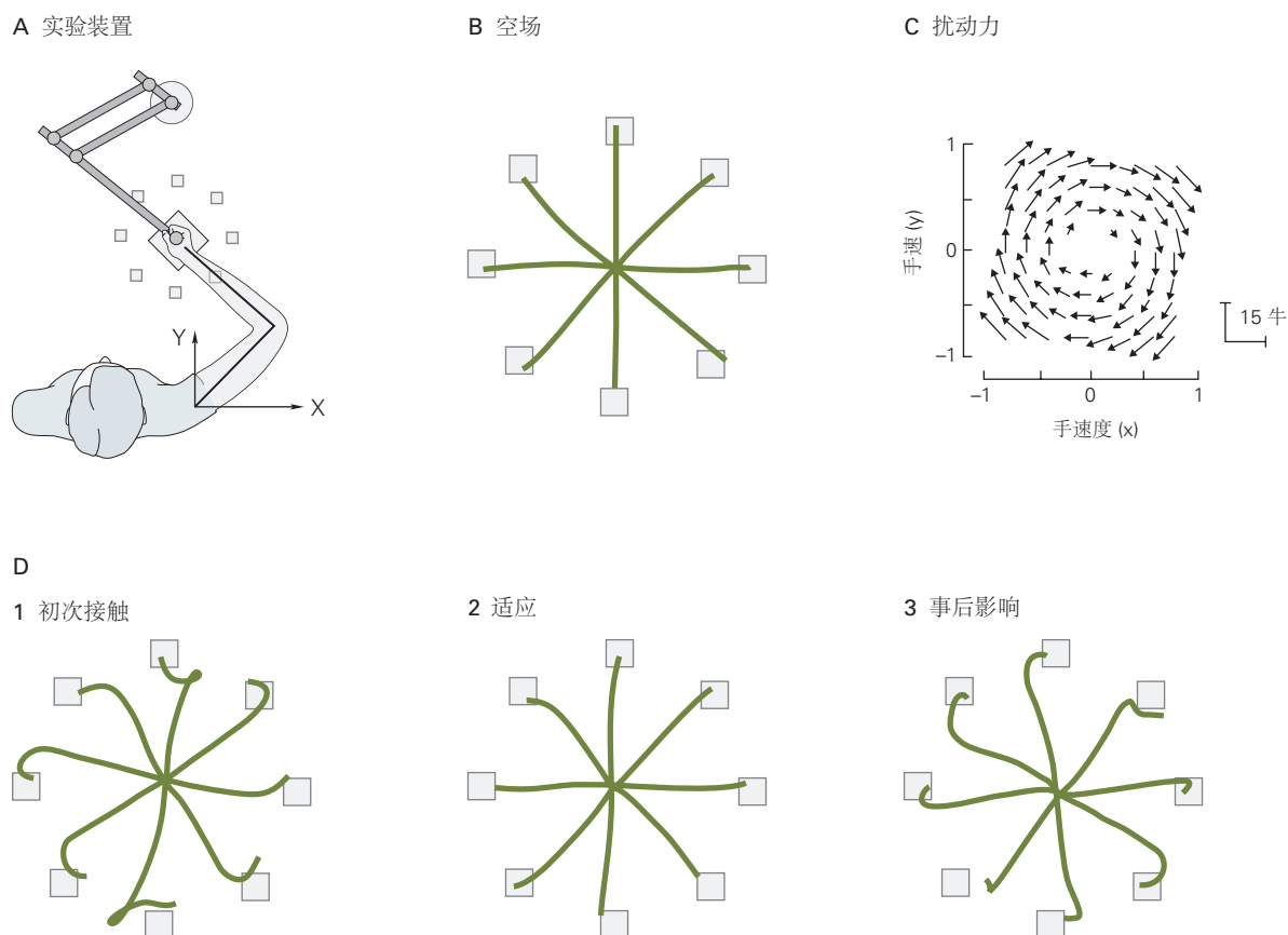
图 30.6.1: 学习提高了在新的动态环境中到达的准确性 [254] 。A. 受试者拿着一个机器人装置，该装置测量手的位置和速度并向手施加力。B. 当运动关闭时（空场），受试者从工作区中心大致直线移动到排列成圆圈的目标。C. 然后向手施加顺时针方向的力，显示为手速度的函数。该场产生与手的速度成正比的力，该力始终与当前运动方向成直角。D. 最初，手的路径受到扰动力（1）的响应而受到严重扰动。一段时间后，受试者适应并可以在整个运动过程中再次沿着直线路径移动（2）。当运动随后关闭时，运动再次受到扰动，但方向与先前的扰动相反（3）。
