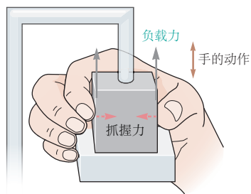
图 30.4.5: 对自发动作的超前控制 [250] 。A. 当指示受试者握住以机械方式施加正弦负载力的物体时，手指的抓握力很高以防止滑动，并且抓握力调节滞后于负载力的变化。其中以深红色实线突出显示的是负载力调节的一部分，这会导致深红色虚线所示的相应抓握力滞后（试验时长为 4 秒）。B. 当受试者通过下拉固定物体产生类似的负载曲线时，可以预期负载力，因此，抓握力较低并且跟踪负载力没有延迟。
