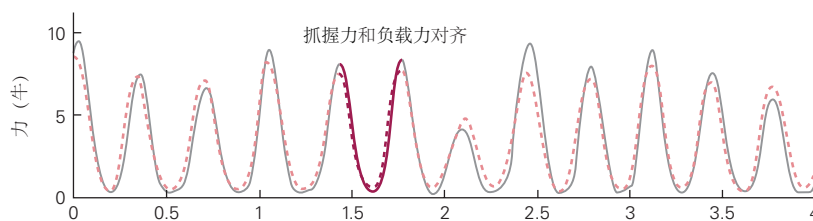
图 30.4.5: 对自发动作的超前控制 [250] 。A. 当指示受试者握住以机械方式施加正弦负载力的物体时，手指的抓握力很高以防止滑动，并且抓握力调节滞后于负载力的变化。其中以深红色实线突出显示的是负载力调节的一部分，这会导致深红色虚线所示的相应抓握力滞后（试验时长为 4 秒）。B. 当受试者通过下拉固定物体产生类似的负载曲线时，可以预期负载力，因此，抓握力较低并且跟踪负载力没有延迟。
