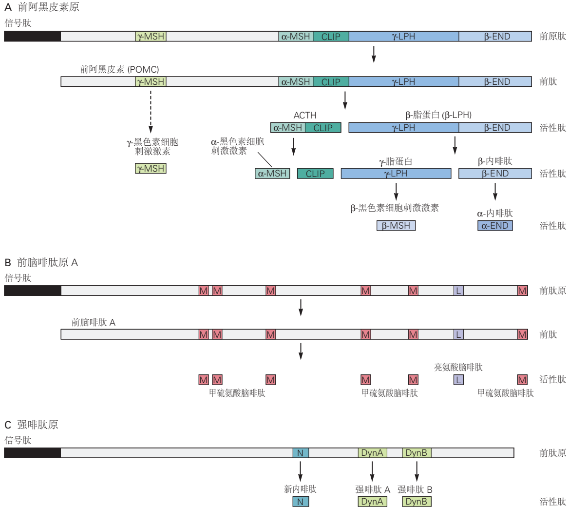
图 16.4.1: 激素和神经肽前体的处理方式不同：神经肽的阿片类药物家族。阿片类神经肽源自较大的前体分子，需要多轮蛋白酶介导的裂解。这些前体经过不同的处理以产生其特定的肽产品。这些前体通过内质网膜的转运是由疏水信号序列启动的。内部切割通常发生在多肽内的碱性残基处。此外，这些前体具有在其加工和功能中发挥作用的关键半胱氨酸残基和糖部分。通常，处理的第一次迭代从新合成的多蛋白前体（称为前肽形式）开始。氨基末端信号序列的切割产生较小的分子，即前肽。3 种主要的阿片肽前体蛋白由 3 个基因编码：前阿黑皮素、前脑啡肽和前强啡肽（未显示）。3 种合成前肽的差异加工产生了主要的阿片肽：内啡肽、脑啡肽和强啡肽。 A. 前阿黑皮素前体在垂体的不同叶中以不同方式加工，产生 \alpha -促黑色素细胞激素和 \gamma -黑色素细胞刺激激素、促皮质激素样中间肽和 \beta -促脂素。 \beta -促脂素被裂解产生 \gamma -促脂素和 \beta -内啡肽，它们本身分别产生 \beta -黑色素细胞刺激激素（ \beta -黑色素细胞刺激激素）和 \alpha -内啡肽。促肾上腺皮质激素和 \beta -促脂素内的内切蛋白水解裂解发生在中叶，而不是前叶。 B. 类似的原理在脑啡肽前体的加工中很明显，它产生了 6 种 Met-脑啡肽和一种 Leu-脑啡肽。 C. 强啡肽前体被切割成至少 3 种与亮氨酸脑啡肽相关的肽，因为所有 3 种肽的氨基末端序列都含有亮氨酸脑啡肽的序列。
