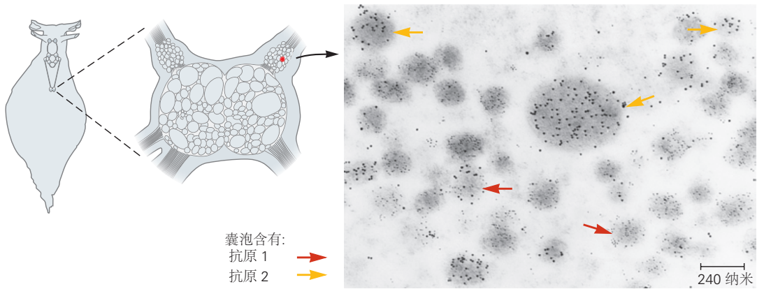
图 16.3.3: 与抗体相连的电子不透明金颗粒用于在超微结构水平上定位组织中的抗原。电子显微照片显示了穿过海兔袋细胞的细胞体的截面。囊细胞通过释放一组从产卵激素前体切割而来的神经肽来控制生殖行为。细胞含有几种致密的核囊泡。用针对产卵激素前体的不同区域中所含的不同氨基酸序列的 2 种抗体处理此处显示的细胞。一种抗体在兔子身上产生，另一种在大鼠身上产生。用山羊饲养的抗兔或抗大鼠免疫球蛋白（第二抗体）检测这些抗体。每种二级抗体都与不同大小的胶体金颗粒偶联。由抗原 1 鉴定的囊泡（用较小的金颗粒标记）小于由抗原 2 鉴定的囊泡（用较大的金颗粒标记），这表明从前体切割的特异性片段定位在不同的囊泡中。
