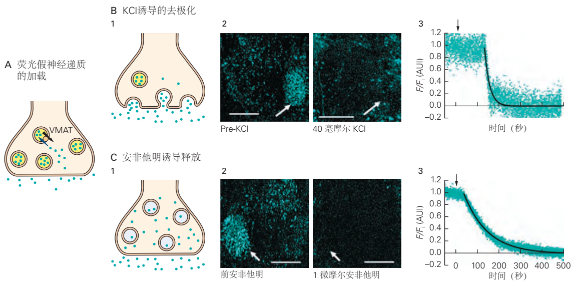
图 16.3.4: 荧光假神经递质标记允许对神经递质释放进行光学监测。A. 荧光假神经递质（蓝点）由囊泡单胺转运蛋白转运到多巴胺神经末梢的突触小泡中。稳定状态下的囊泡呈酸性，如黄色阴影所示。B. 1. 提高细胞外 KCl 浓度导致去极化并通过胞吐作用释放囊泡，导致荧光标记丢失（脱色）。2. KCl（40 毫摩尔）去极化导致突触前多巴胺神经末梢的荧光假神经递质 206 快速脱色。用荧光假神经递质 206（300 纳摩尔）将整个果蝇大脑加载到稳定状态，并用 KCl 处理。在 KCl 诱导的去极化之前（左）和之后（右）神经细胞的投射图像堆栈。3. 代表性实验的荧光衰减动力学。黑色箭头表示开始添加 KCl。比例尺 = 25 微米。C. 1. 苯丙胺通过文中讨论的非胞吐机制导致囊泡脱酸（黄色阴影消失）及其脱色。2. 苯丙胺（1 微摩尔）导致荧光假神经递质 206 脱色。用荧光假神经递质 206（300 纳摩尔）将整个果蝇大脑加载到稳定状态，并用苯丙胺处理。治疗前（左）和治疗后（右）神经细胞的投射图像堆栈。3. 代表性实验的荧光衰减动力学。黑色箭头表示开始添加药物。比例尺 = 25 微米。
