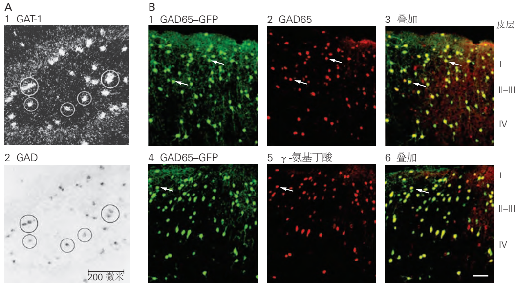
图 16.3.2: 可视化化学信使的技术。A. 大鼠海马体的光学显微镜切片。1. 使用编码 \gamma -氨基丁酸转运蛋白 GAT-1 的信使核糖核酸的探针的原位杂交。用 \alpha - 35 S dATP 对探针进行末端标记, 并通过覆盖的放射自显影照相乳剂中的银颗粒簇进行观察。2. 用与碱性磷酸酶连接的寡核苷酸探针对谷氨酸脱羧酶的信使核糖核酸进行原位杂交, 谷氨酸脱羧酶是 \gamma -氨基丁酸的特异性生物合成酶。谷氨酸脱羧酶探针通过细胞质中有色碱性磷酸酶反应产物的积累而显现。表达 GAT-1 和谷氨酸脱羧酶转录物的神经元分别用银粒和磷酸酶反应标记, 并用包含这 2 种标记的细胞体周围的圆圈表示。B. 来自谷氨酸脱羧酶 65-绿色荧光蛋白转基因小鼠的新皮层的图像, 其中绿色荧光蛋白在谷氨酸脱羧酶 65 启动子的控制下表达。绿色荧光蛋白与谷氨酸脱羧酶 65 (1-3) 和 \gamma -氨基丁酸 (4-6) (均通过间接免疫荧光检测) 共同定位于不同层的神经元中。大多数绿色荧光蛋白阳性神经元对谷氨酸脱羧酶 65 和 \gamma -氨基丁酸呈免疫阳性 (箭头显示所选实例)。比例尺 = 100 微米。
