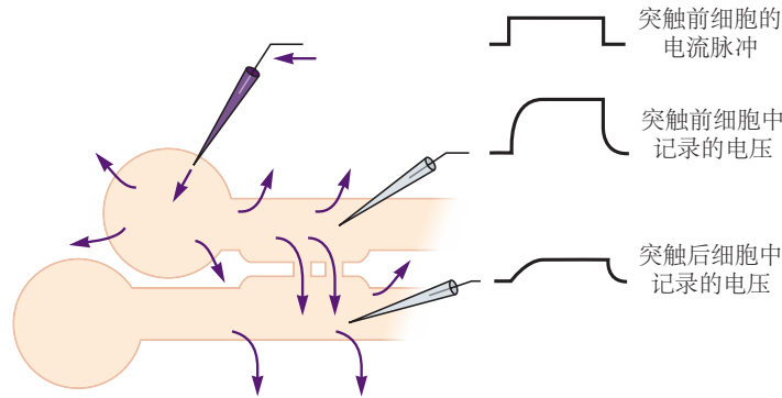
图 11.2.3: 电传输是分级的。即使突触前细胞中的电流低于动作电位的阈值，它也会发生。如单细胞记录所示，亚阈值去极化刺激会导致突触前和突触后细胞发生被动去极化（去极化或外向电流由向上偏转表示）。
