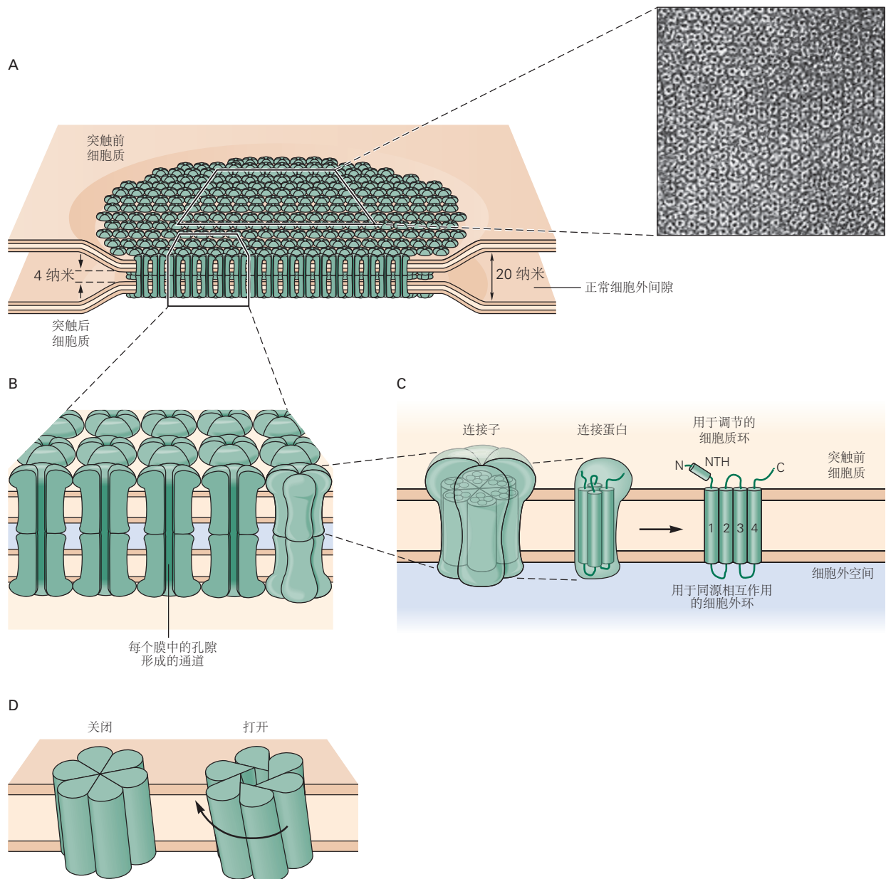
图 11.2.4: 基于 X 射线和电子衍射研究的间隙连接通道的三维模型。A. 电突触或间隙连接由许多跨越突触前和突触后神经元膜的专门通道组成。这些间隙连接通道允许电流直接从一个细胞传递到另一个细胞。电子显微照片中的通道阵列是从已经过负染色的大鼠肝细胞膜中分离出来的，这种技术使通道周围和空隙中的区域变暗。每个通道的轮廓都是六角形的。放大 307,800 倍。B. 间隙连接通道实际上是一对半通道，每个对应细胞中都有一个连接 2 个细胞的细胞质 [63] 。C. 每个半通道或连接子由 6 个相同的亚基（称为连接蛋白）组成。每个连接蛋白长约 7.5 纳米，跨越细胞膜。单个连接蛋白具有细胞内 N 端和 C 端，包括短的细胞内 N 端 \alpha 螺旋（NTH）和 4 个跨膜 \alpha 螺旋（1-4）。来自许多不同种类组织的间隙连接蛋白的氨基酸序列具有相似区域（包括跨膜螺旋和细胞外区域），它们参与适当半通道的同嗜性匹配。D. 连接蛋白的排列方式是在结构的中心形成一个孔。由此产生的连接子，孔径约为 1.5 至 2 纳米，具有特征性的六边形轮廓，如 A 部分的照片所示。在一些间隙连接通道中，当亚基在细胞质基部顺时针方向旋转约 0.9 纳米时，孔就会打开 [64] 。
