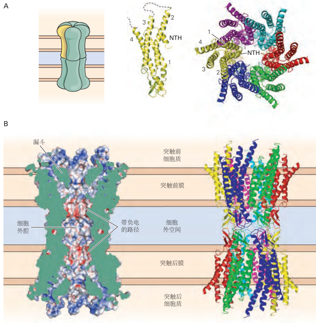
图 11.2.5: 间隙连接通道的高分辨率三维结构。所有结构均由人连接蛋白 26 亚基形成的间隙连接通道的 X 射线晶体学确定。 A. 左图：完整的间隙连接通道图，显示了一对并列的半通道。中图：单个连接蛋白亚基的高分辨率结构显示 4 个跨膜 \alpha 螺旋 (1-4) 和一个短的 N 末端螺旋 (NTH)。亚基的方向对应于右图中黄色亚基的方向。右图：从细胞质观察半通道的自下而上视图。6 个亚基中的每一个都有不同的颜色。黄色亚基的螺旋被编号。方向对应于左图中黄色半通道的方向，向观察者旋转 90 度。 B. 膜平面中间隙连接通道的 2 个侧视图显示 2 个并列的半通道。方向与 A 部分相同。左：通过通道的横截面显示通道孔的内表面。蓝色表示带正电的表面；红色表示带负电的表面。细胞质入口（漏斗）孔内的绿色物质被认为代表由 N 端螺旋形成的通道门。右图：通道的侧视图以与 A 部分相同的配色方案显示了 6 个连接蛋白亚基中的每一个。整个间隙连接通道大约 9 纳米宽 \times 15 纳米高。
