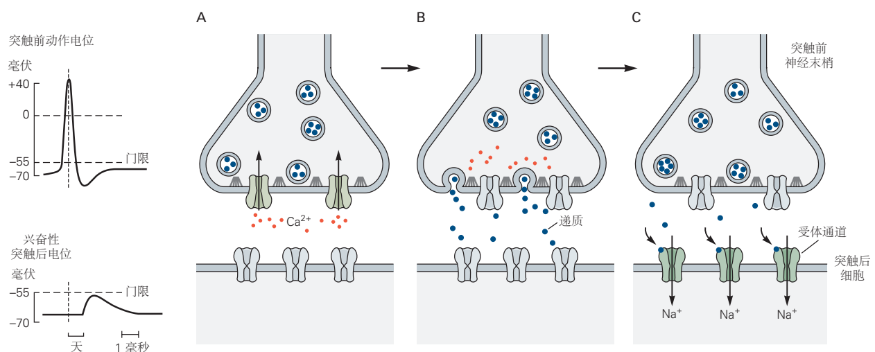
图 11.2.2: 化学突触的突触传递涉及几个步骤。如图 11.2.1B 所示，与电突触处几乎瞬时的信号传递相比，化学突触传递的复杂过程解释了突触前细胞中的动作电位与突触后细胞中的突触电位之间的延迟。A. 到达突触前轴突末端的动作电位导致活动区的电压门控 \text{Ca}^{2+} 通道打开。灰色细丝代表活性区的对接和释放位点。B. \text{Ca}^{2+} 通道开放活性区附近产生高浓度的细胞内 \text{Ca}^{2+} ，导致含有神经递质的囊泡与突触前细胞膜融合并将其内容物释放到突触间隙（称为胞吐作用的过程）。C. 释放的神经递质分子然后扩散到突触间隙并结合突触后膜上的特定受体。这些受体导致离子通道打开（或关闭），从而改变突触后细胞的膜电导和膜电位。
