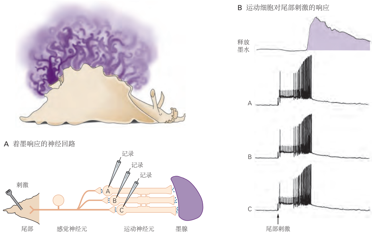
图 11.2.6: 一起放电的电耦合运动神经元可以产生同步行为 [65] 。A. 在海螺海兔中，来自尾部神经节的感觉神经元与支配墨腺的 3 个运动神经元形成突触。运动神经元通过电突触相互连接。B. 应用于尾部的一系列刺激会在所有 3 个运动神经元中产生同步放电，从而导致墨水释放。
