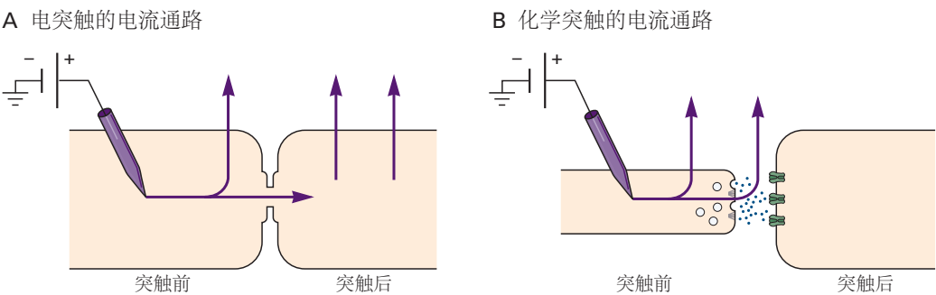
图 11.1.1: 电突触和化学突触的功能特性。A. 在电突触处, 一些注入突触前细胞的电流通过细胞膜中的静息（非门控）离子通道逸出。然而, 一些电流也通过间隙连接通道进入突触后细胞, 间隙连接通道连接突触前细胞和突触后细胞的细胞质, 并为电流提供低电阻（高电导）通路。B. 在化学突触处, 所有注入突触前细胞的电流都会逃逸到细胞外液中。然而, 由此产生的突触前细胞膜去极化会产生动作电位, 导致释放与突触后细胞上的受体结合的神经递质分子。这种结合打开离子通道, 引发突触后细胞膜电位的变化。
