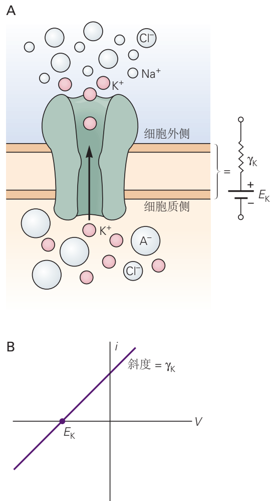
图 9.5.1: 化学力和电力有助于电流通过离子通道。A. K^+ 的浓度梯度会产生电动势，其值等于 E_K ，即 K^+ 的能斯特电势。这可以用细胞来表示。在该回路中，细胞 E_K 与导体 \gamma_K 串联，代表 K^+ 通道的电导。B. 在电驱动力和化学驱动力同时存在的情况下， K^+ 通道的电流-电压关系。电流为 0 时的膜电位等于 K^+ 能斯特电位。
